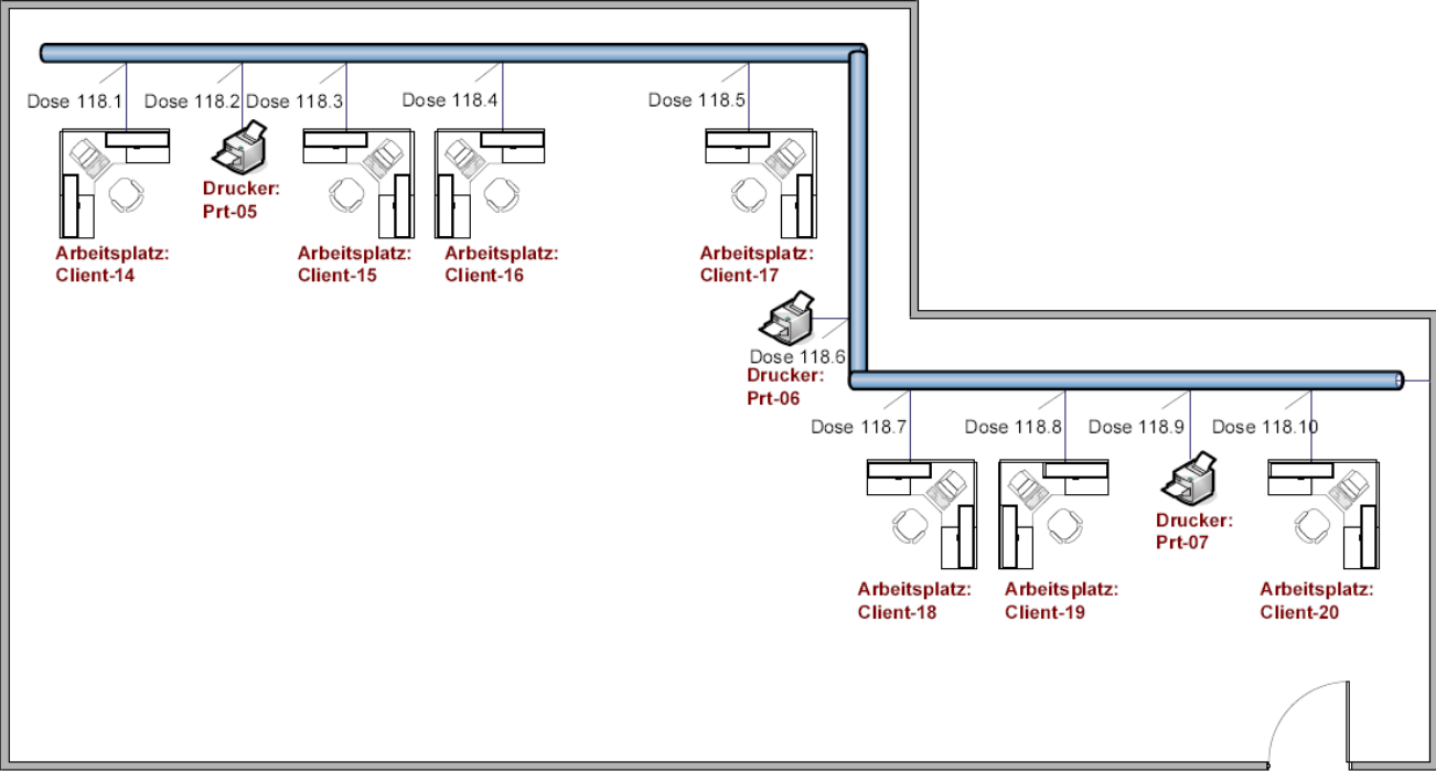
Netzwerkplan 1. Etage, Zi. 118, Mustermann AG, Hansdorf
